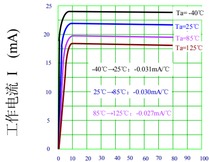
V-I 温度特性(典型)
