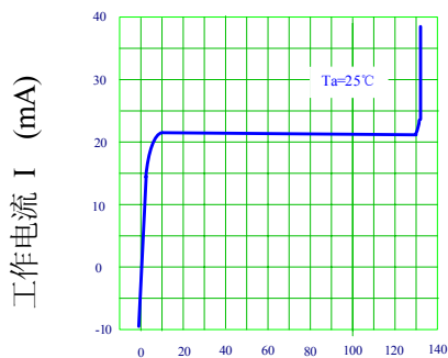
V-I 输出特性(典型)
