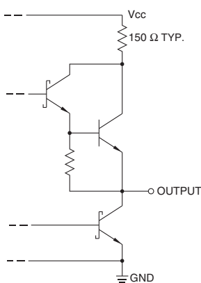
74OL6000/01 Output
