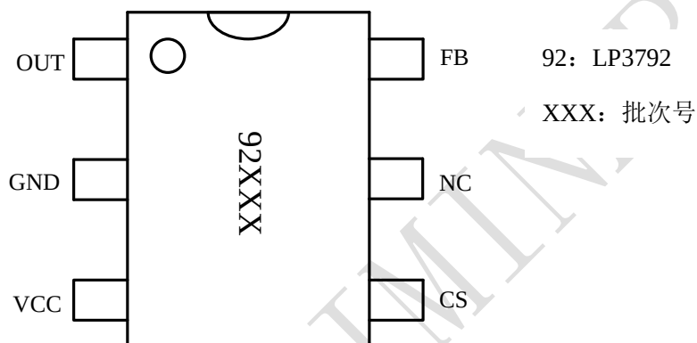
图 2 管脚封装图
